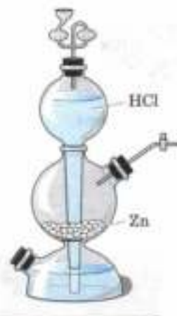
Рис. 53. Аппарат Киппа
