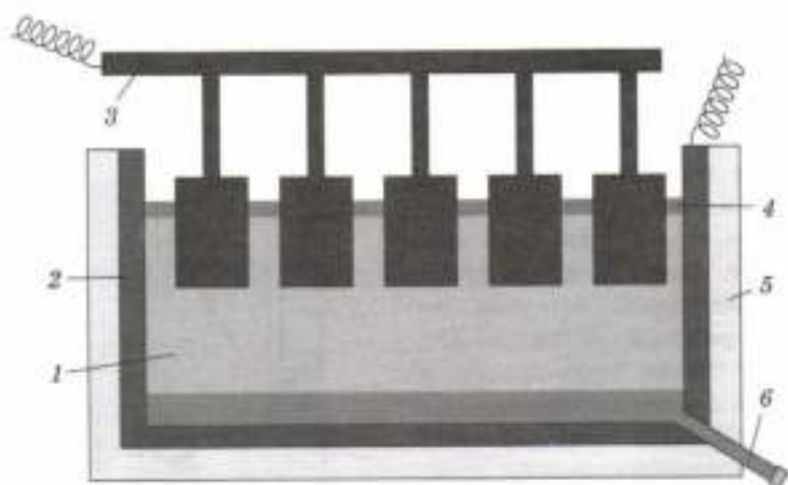
Рис. 112. Схема установки для промышленного получения алюминия: 1 — электролит — расплавленный криолит с добавками фторидов кальция и алюминия (для снижения температуры плавления) и оксид алюминия (добавляют периодически); 2 — угольный катод; 3 — угольный анод; 4 — корка из застывшего оксида алюминия, защищающая расплавленный алюминий от окисления; 5 — стальная ванна; 6 — отбор расплавленного алюминия
