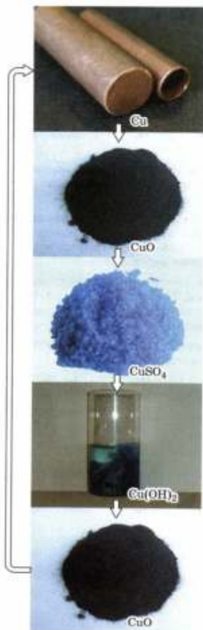
Рис. 147. Генетический ряд меди
