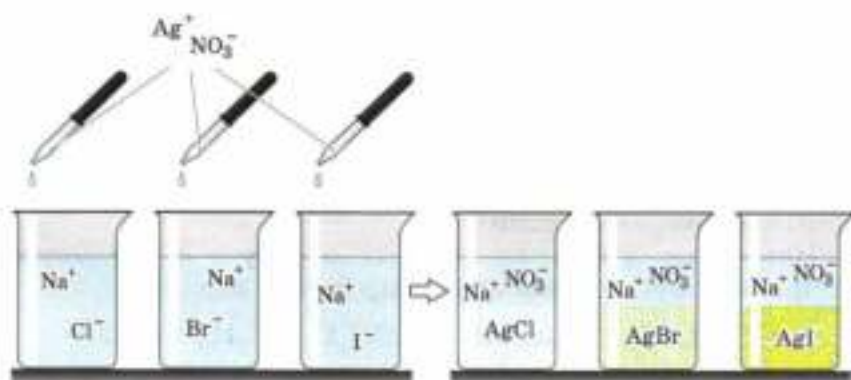
Рис. 132. Качественные реакции на галогенид-анионы: хлорид-анион, бромид-анион, иодид-анион
