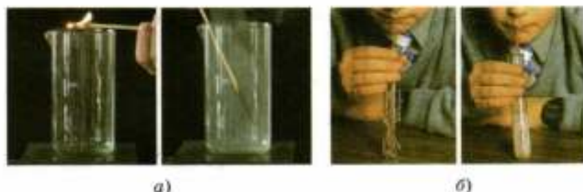
Рис. 63. Способы распознавания углекислого газа: а — тлеющей лучинкой; б — известковой водой
