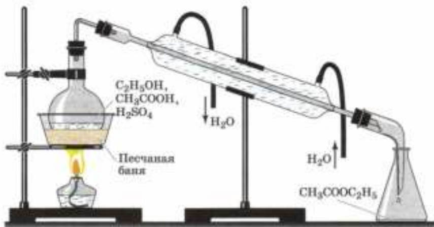
Рис. 134. Прибор для получения уксусно-этилового эфира
