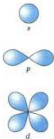
Рис. 3. Формы s -, p -, d -электронных облаков
