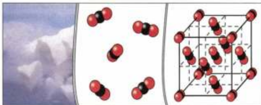
Рис. 9. Углекислый газ — это вещество с молекулярной кристаллической решёткой
