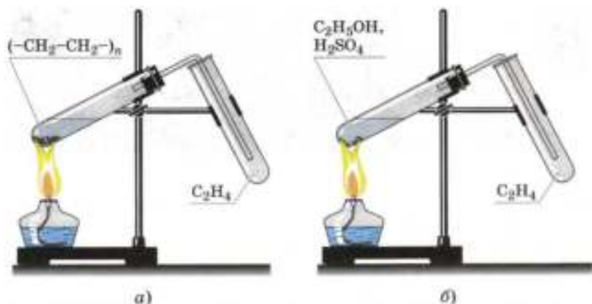
Рис. 67. Лабораторные способы получения этилена: а — деполимеризация полиэтилена; б — каталитическая дегидратация этилового спирта
