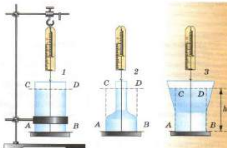
Рис. 110. Гидростатический парадокс
