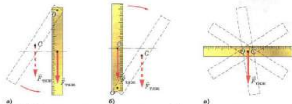
Рис. 188. Расположение центра тяжести при устойчивом равновесии
