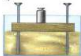
Рис. 90. Зависимость давления от площади опоры
