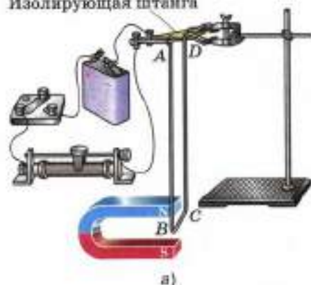
Рис. 101. Действие магнитного поля на проводник с током
