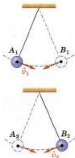
Рис. 60. Колебания маятников, происходящие в противоположных фазах
