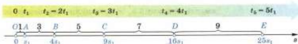
Рис. 15. Закономерности равноускоренного движения: OA : OB : OC : OD : OE = 1 : 4 : 9 : 16 : 25 ; OA : AB : BC : CD : DE = 1 : 3 : 5 : 7 : 9
