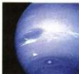
Рис. 182. Большое Тёмное Пятно Нептуна
