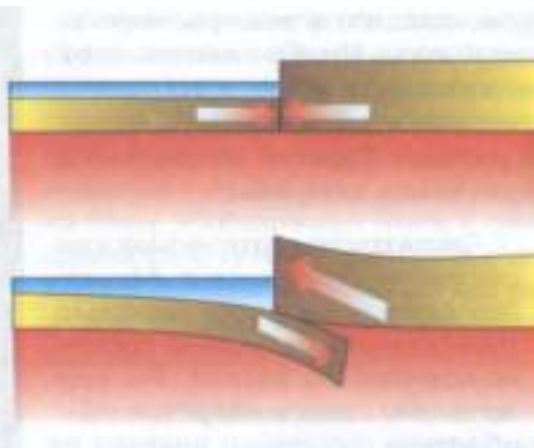
Рис. 24. Столкновение участков материковой и океанической земной коры
