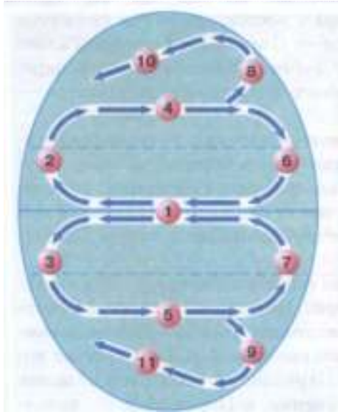
Рис. 54. Схема течений в идеальном океане
