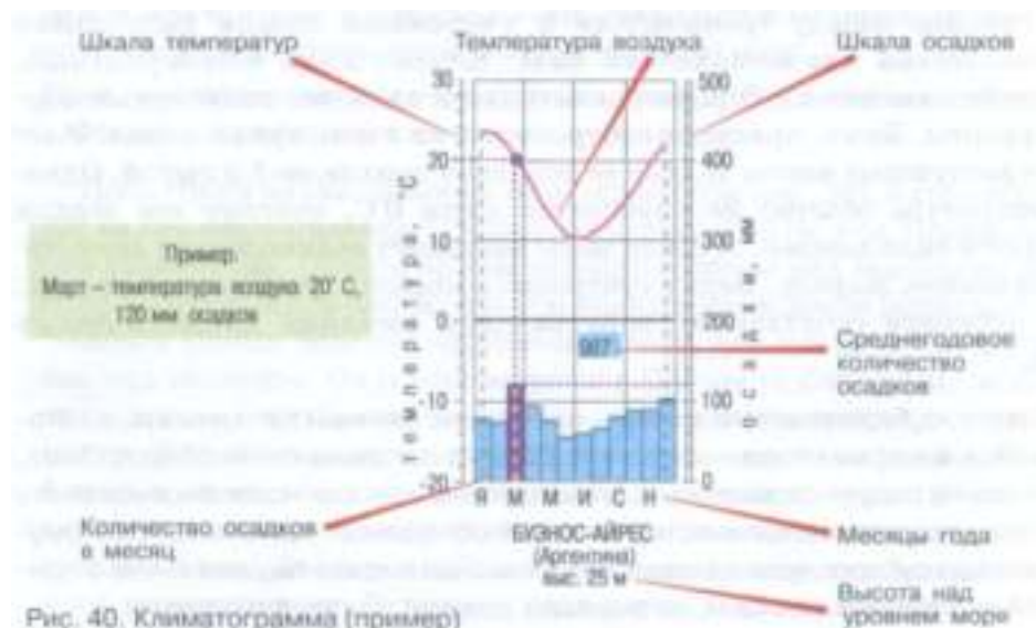
Рис. 40. Климатограмма (пример)
