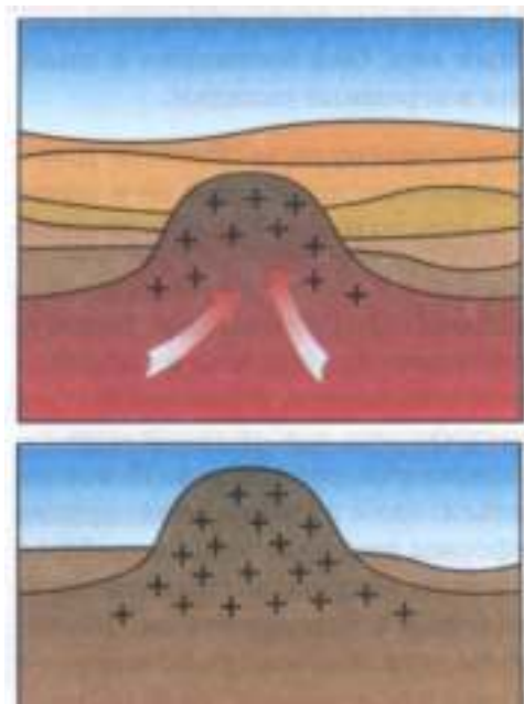
Рис. 31. Образование лакколита
