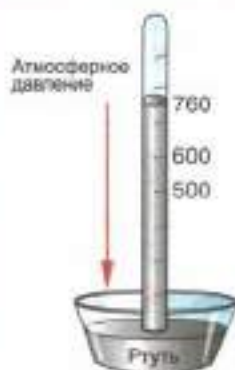
Рис. 115. Опыт Торричелли
