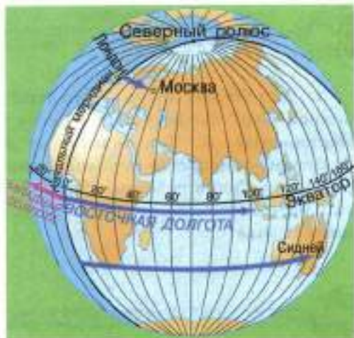
Рис. 40. Географическая долгота
