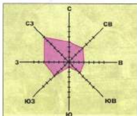
Рис. 122. Роза ветров
