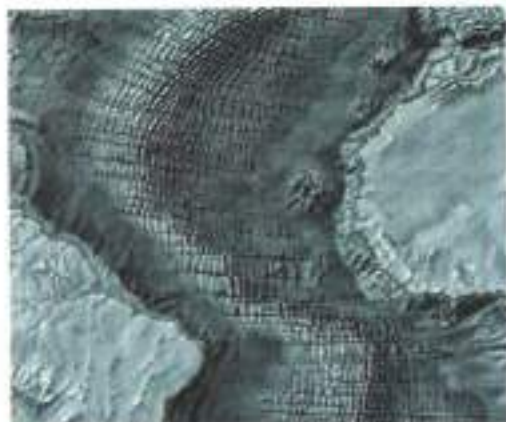
Рис. 102. Срединно-океанический хребет
