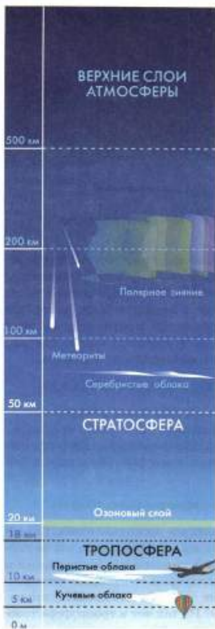
Рис. 106. Строение атмосферы
