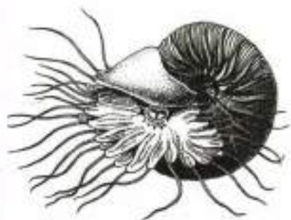
Рис. 80. Аммонит
