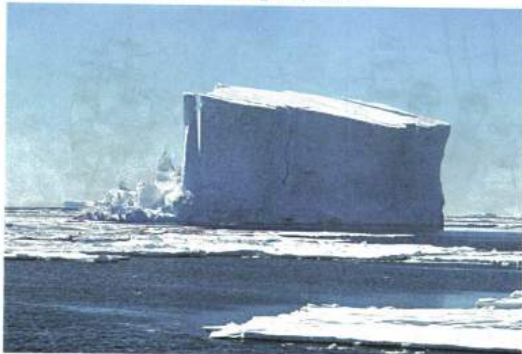
Рис. 18. Айсберг
