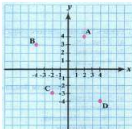
Рис. 37. Математические координаты
