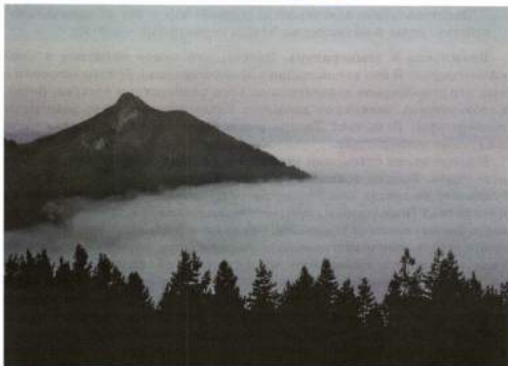
Рис. 124. Туман
