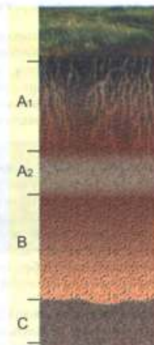
Рис. 101. Почвенные горизонты
