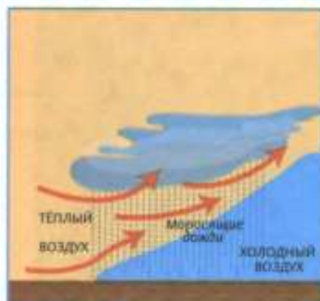
Рис. 61. Тёплый фронт
