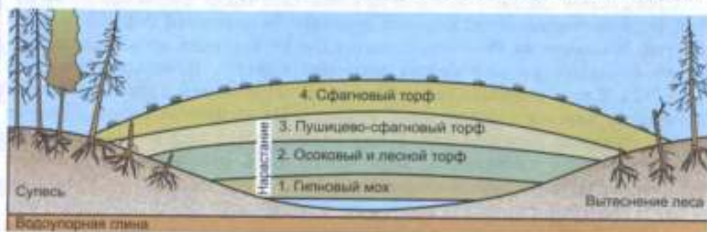
Рис. 83. Верховое болото
