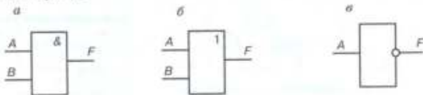
Рис. 1.5. Логические элементы
