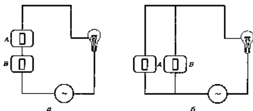
Рис. 1.3. Электрические схемы последовательного (а) и параллельного (б) соединения переключателей
