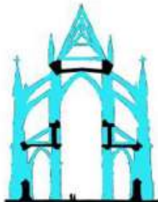
Схема готического храма в разрезе
