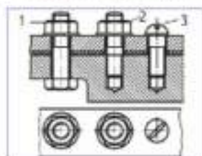
Рис. 6.5. Основные виды резьбовых соединений
