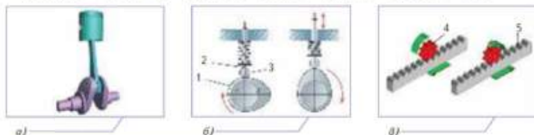
Рис. 4.9. Механизмы передачи и преобразования движения: а — кривошипно-шатунный; б — кулачковый; в — реечный; 1 — кулачок; 2 — шток; 3 — ролик; 4 — колесо; 5 — рейка
