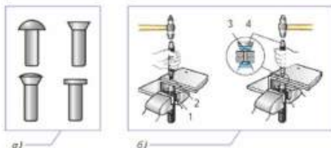
Рис. 6.6. Клейка деталей из металлов и пластмасс: а — виды заклёпок; б — технология клёпки: 1 — натяжка; 2 — поддержка; 3 — замыкающая головка заклёпки; 4 — обжимка
