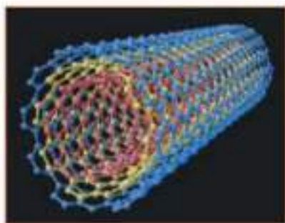
Рис. 14.5. Нанобъекты
