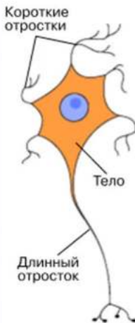
Рис. 93. Строение нейрона
