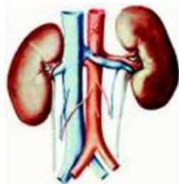
Рис. 80. Почки млекопитающих
