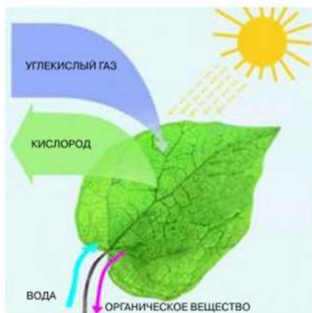
Рис. 60. Фотосинтез
